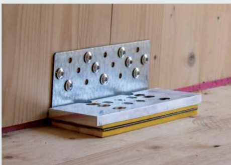
Abb.: Elastischer Winkelverbinder GEPI Connect 240
