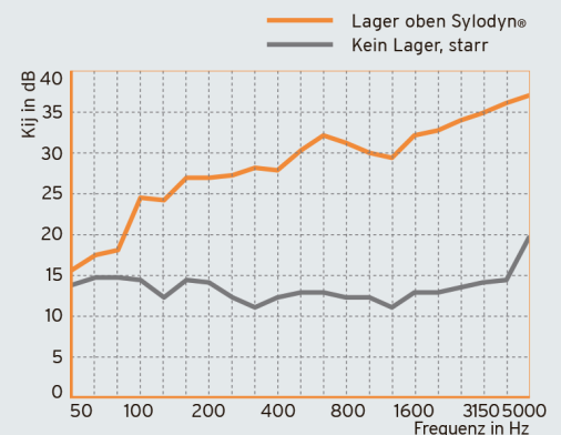
Abb.: Verbesserung des Stoßstellen-dämmmaßes nach EN ISO 10848
