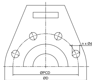
DN 50 - 600 (Design F)
